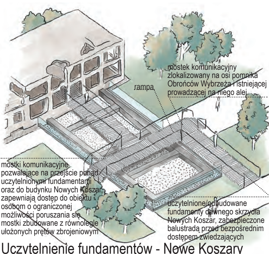
Uczytelnienie fundamentów - Nowe Koszary
